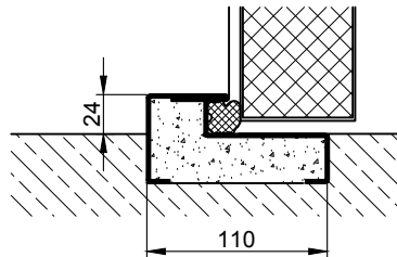
Anschlagschwelle mit Dichtungsprofil
